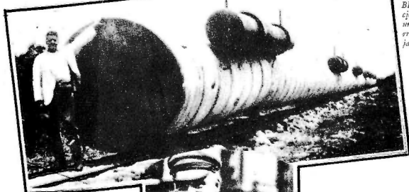
MATANZAS, Cuba. —Una porción del inmenso tubo de tres pies de diámetro que el eminente científico francés GEORGES CLAUDE proyecta sumergir en un tenebroo ensayo en la bahía matanzera, para generar fuerza eléctrica aprovechando los contrastes termales del Golf Stream.
